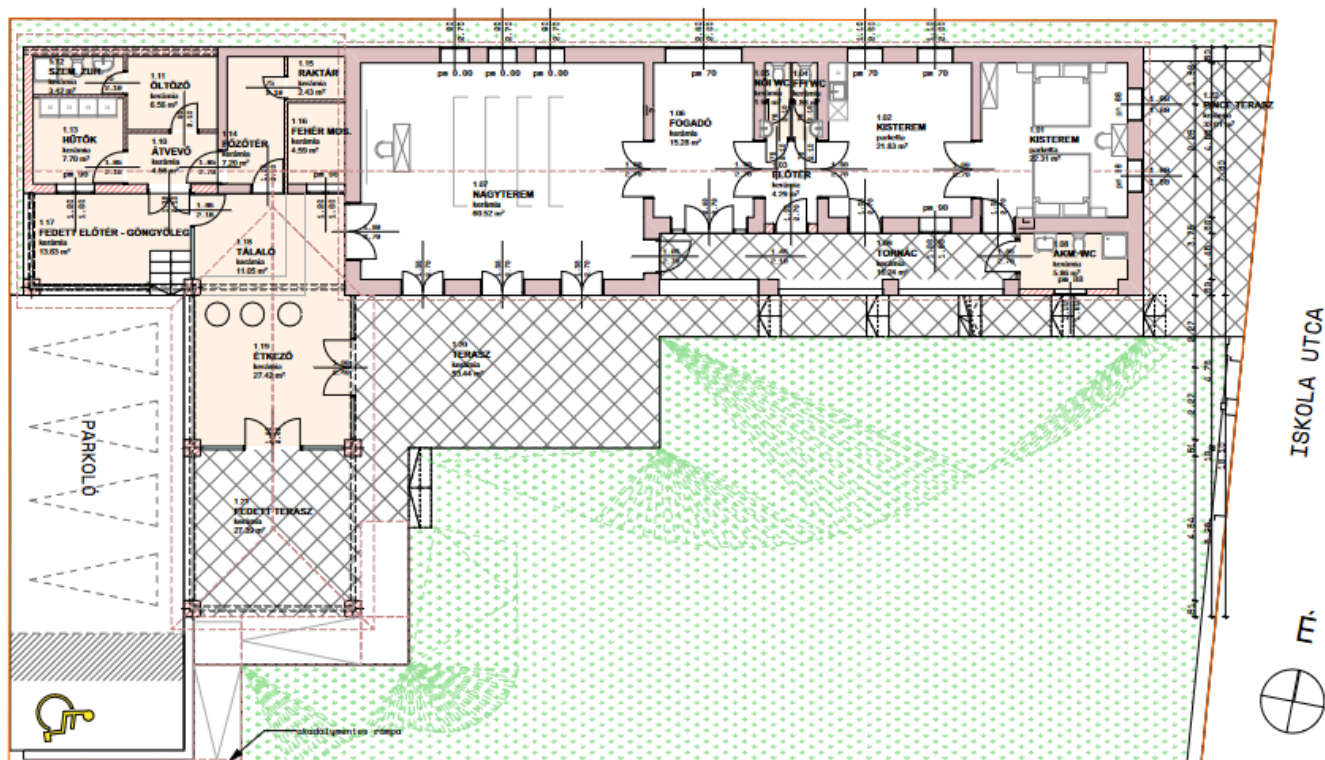
A hosszúhetényi közösségi ház alaprajza (Borbás Gábor terve)
